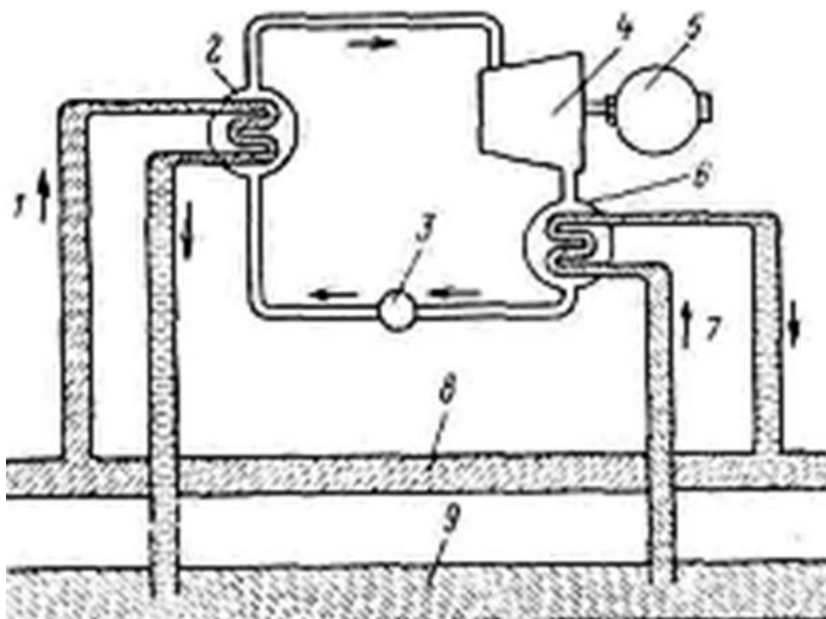
Рисунок 7 Схема преобразования тепловой энергии океана:
