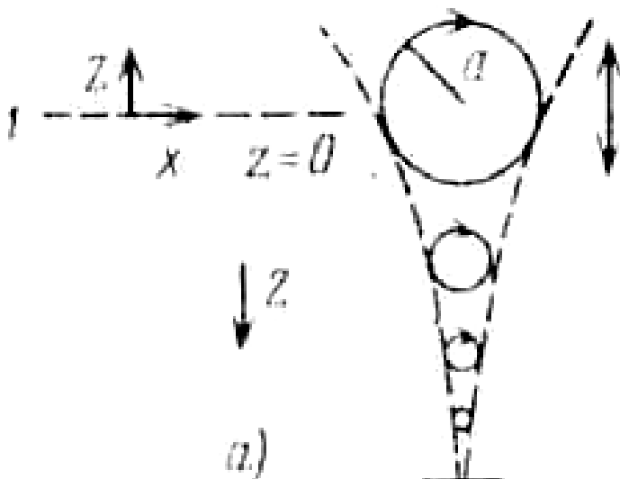
Рисунок 5.1 Определение радиуса круговой орбиты частицы на глубокой воде
